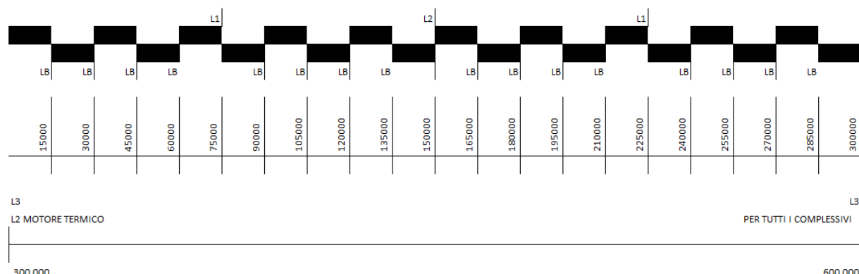
Figura 1: Manutenzione programmata chilometrica delle automotrici Diesel-Elettriche Rimorchiate
